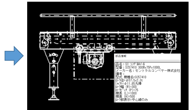
MICRO CADAM図面に取り込まれた部品データと部品情報の表示
